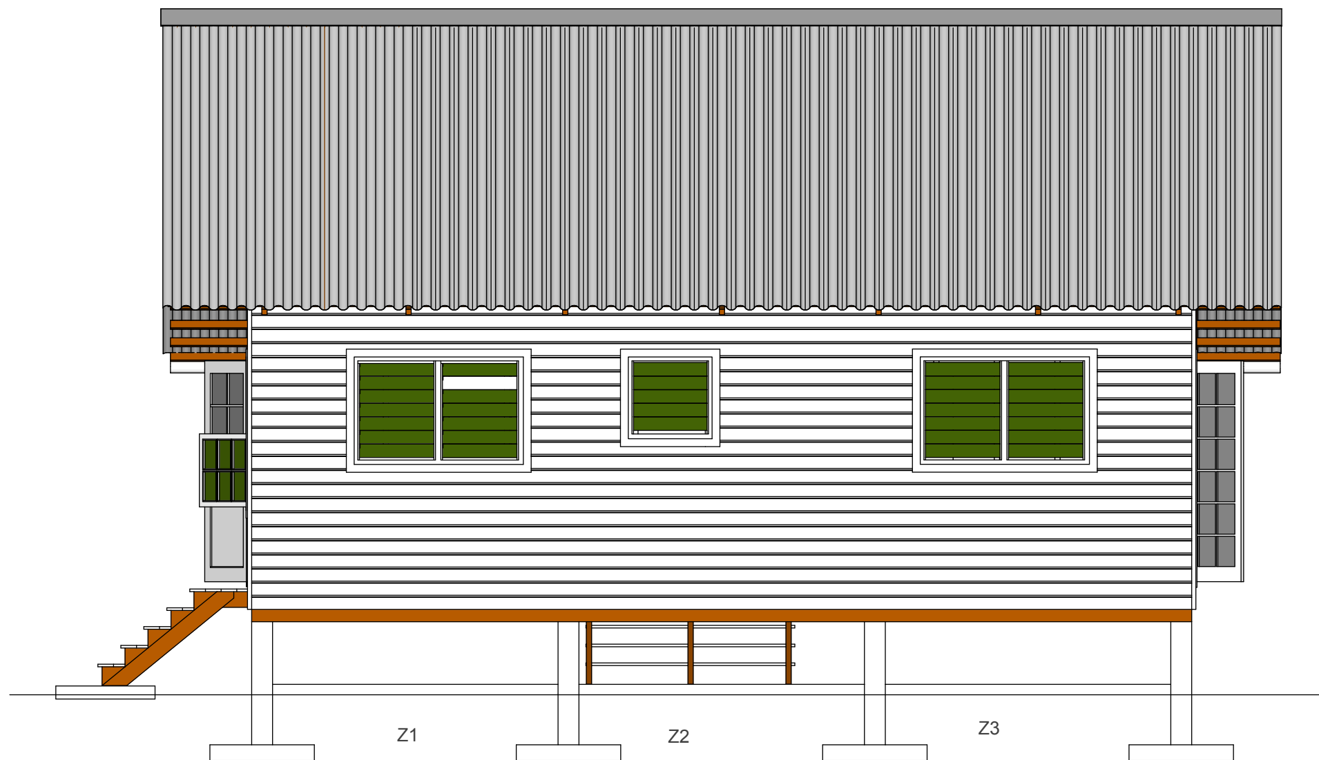
Achter gevel
